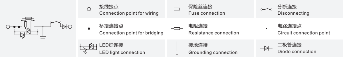
电路图 Circuit diagram
